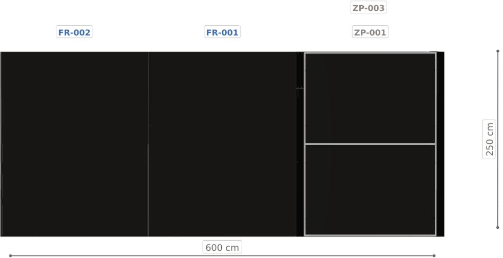
Elewacja tylna
