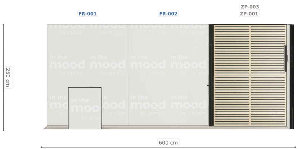
Elewacja frontowa
