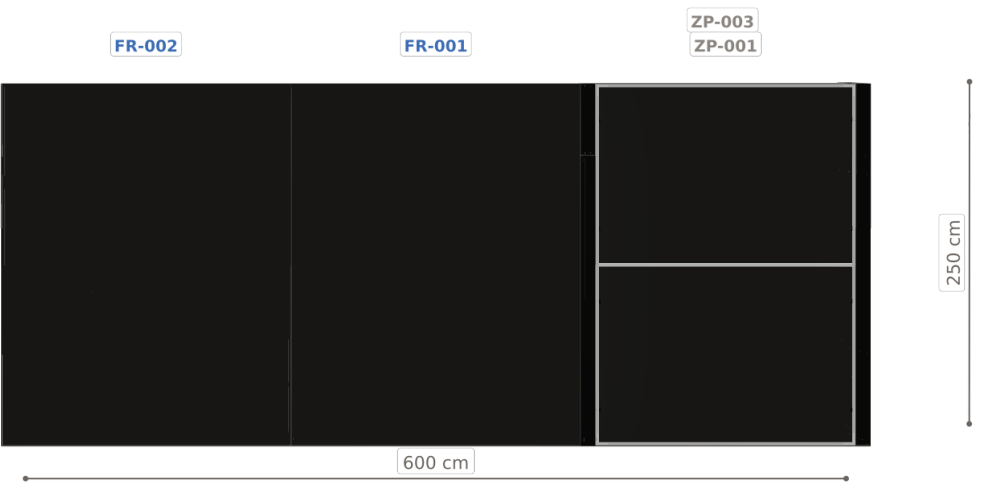
Elewacja tylna
