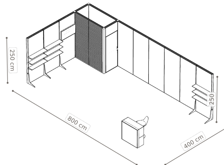
Izometria — wysokości elementów
