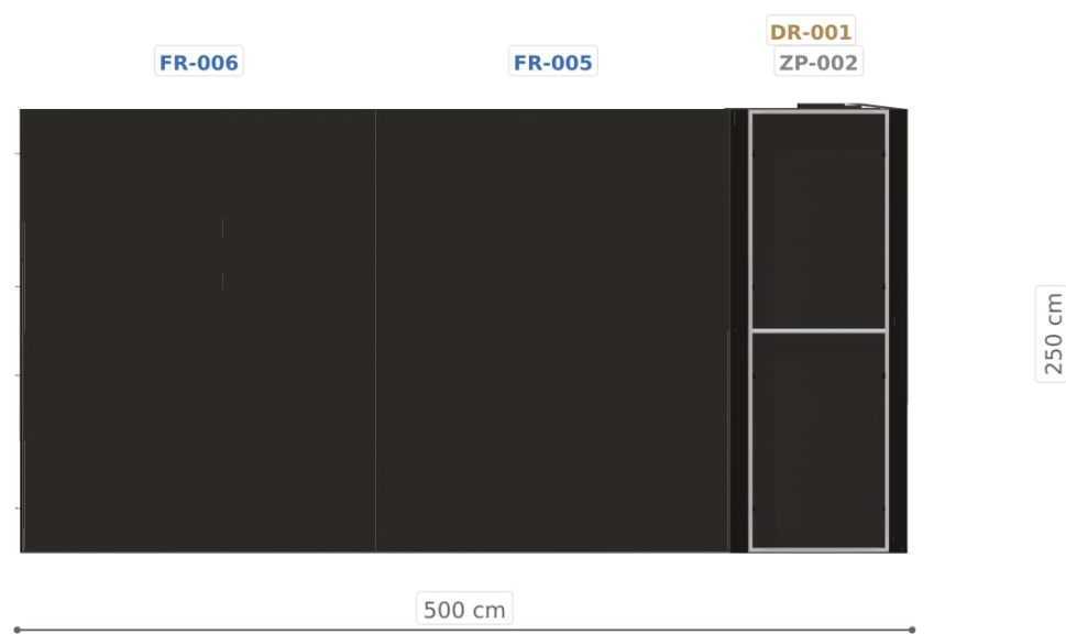
Elewacja tylna
