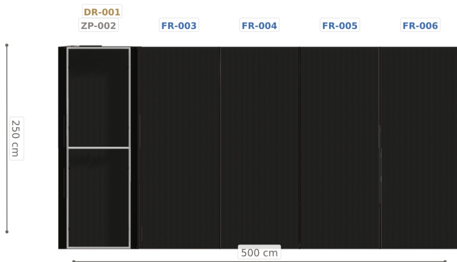
Elewacja frontowa
