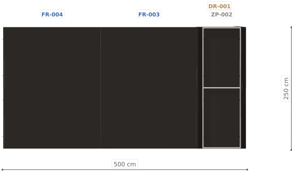
Elewacja tylna
