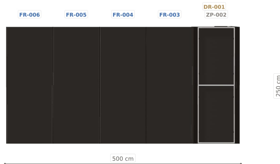
Elewacja tylna
