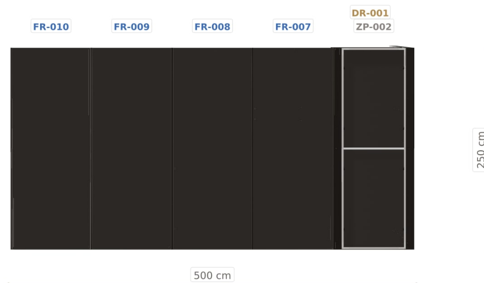
Elewacja prawa
