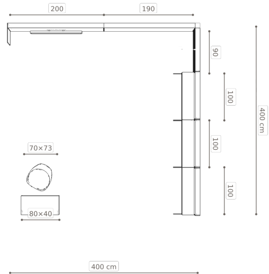
Rzut — szerokości modułów i mebli
