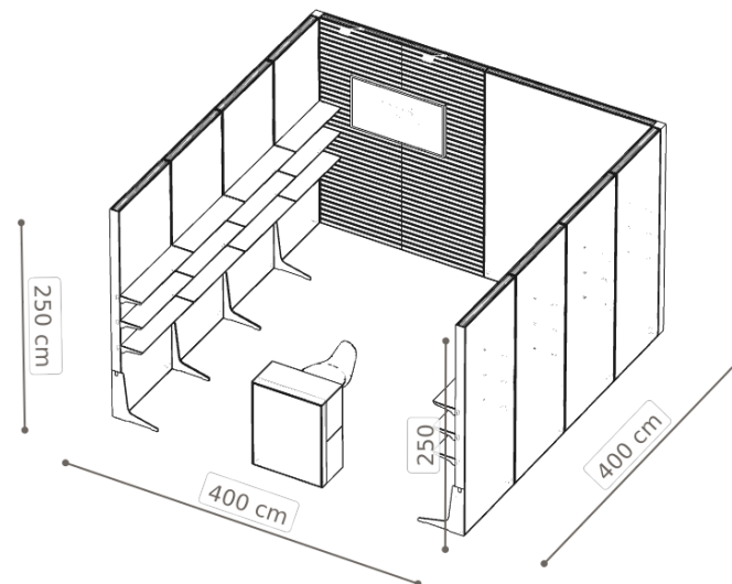
Izometria — wysokości elementów
