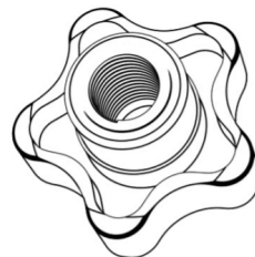
Gałka z gwintem wewnętrznym M6 gałka \varnothing 33 mm
