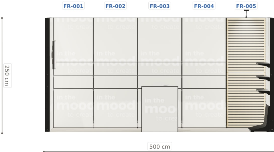
Elewacja frontowa
