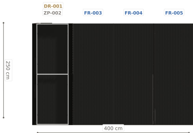
Elewacja frontowa
