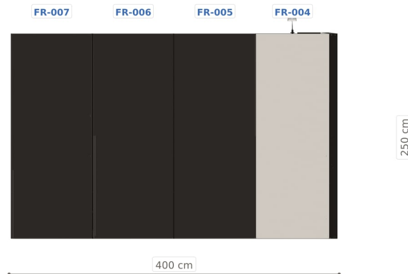
Elewacja prawa
