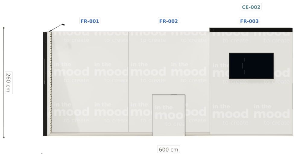
Elewacja frontowa
