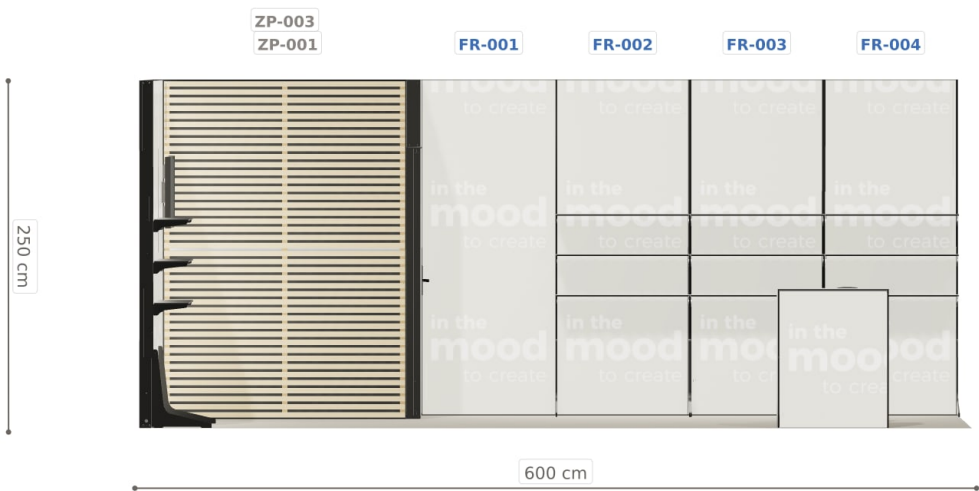
Elewacja frontowa
