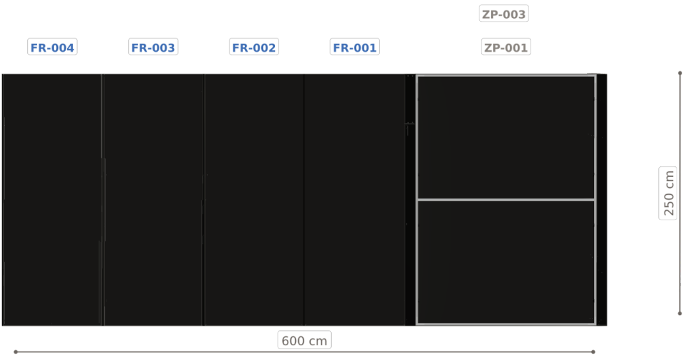
Elewacja tylna
