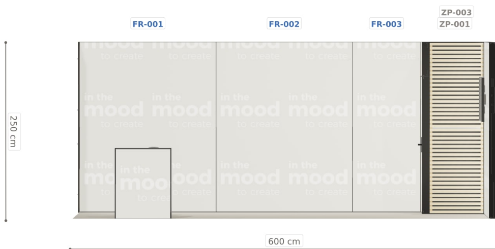
Elewacja frontowa
