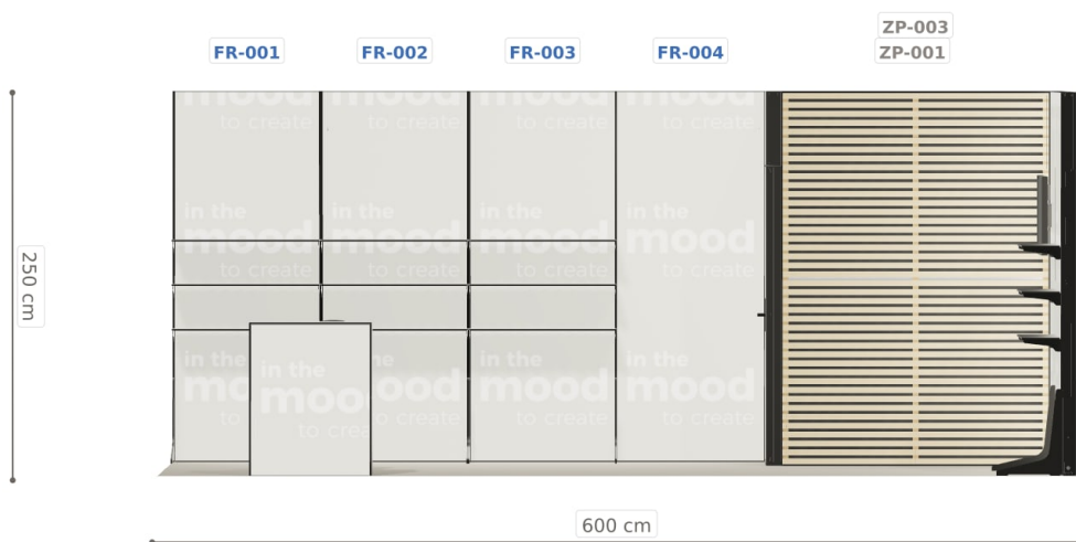
Elewacja frontowa
