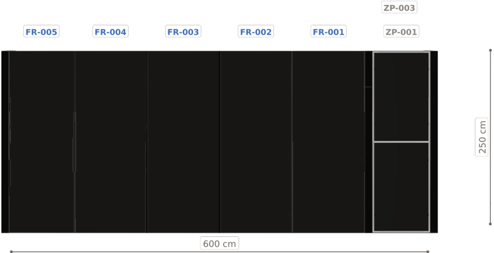
Elewacja tylna
