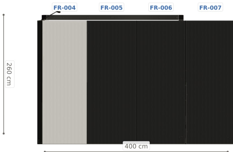
Elewacja frontowa
