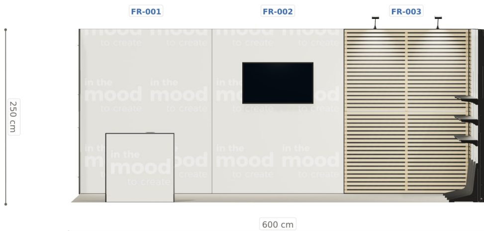
Elewacja frontowa
