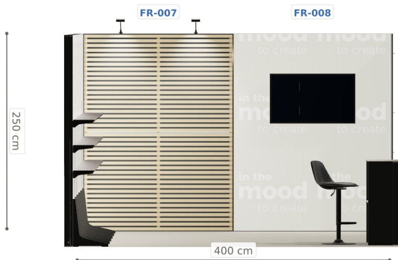
Elewacja lewa
