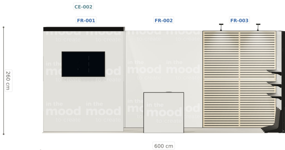
Elewacja frontowa
