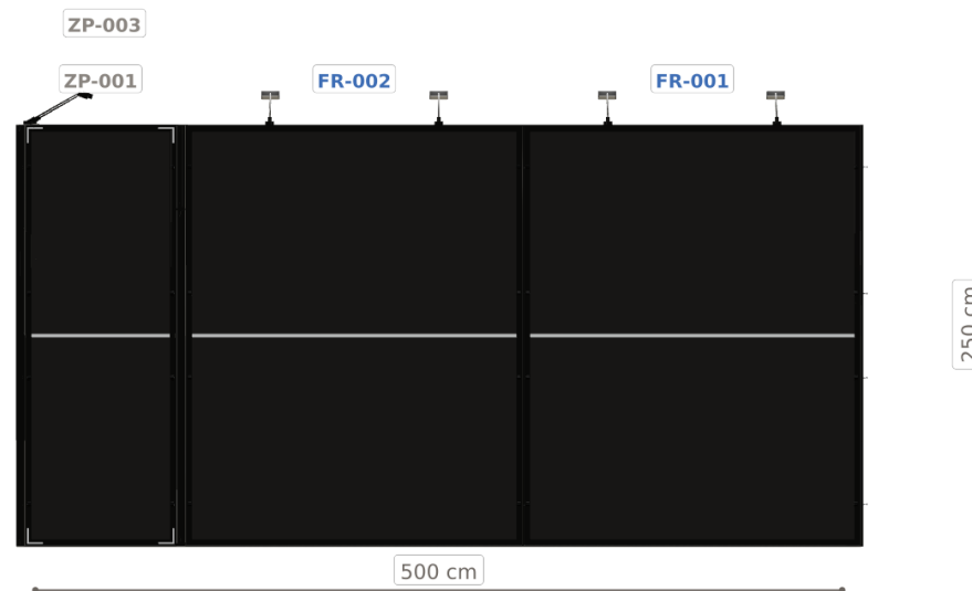
Elewacja tylna
