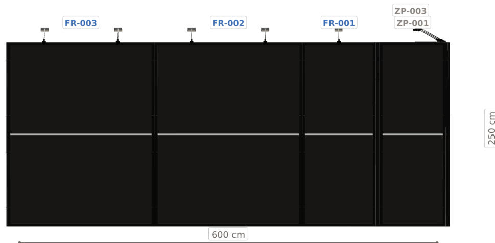
Elewacja tylna
