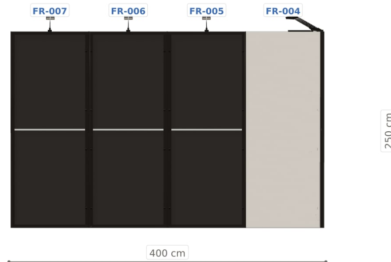
Elewacja tylna
