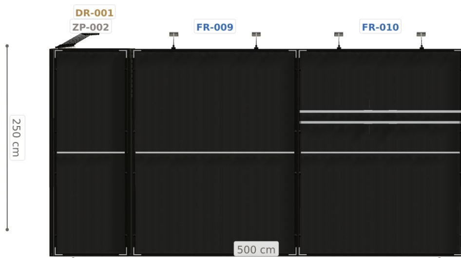
Elewacja lewa
