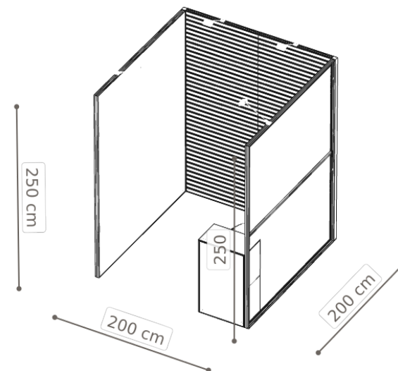
Izometria — wysokości elementów
