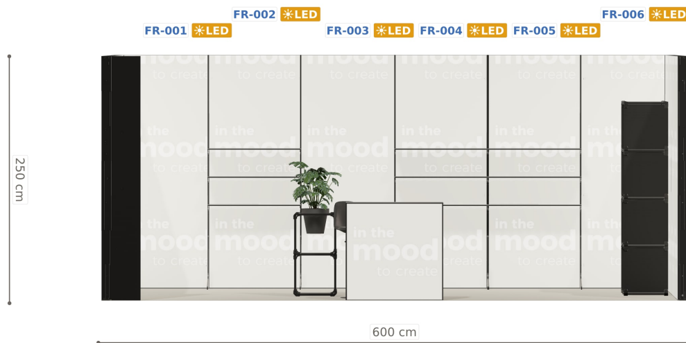
Elewacja ściany tylnej
