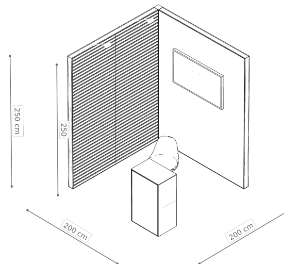
Izometria — wysokości elementów
