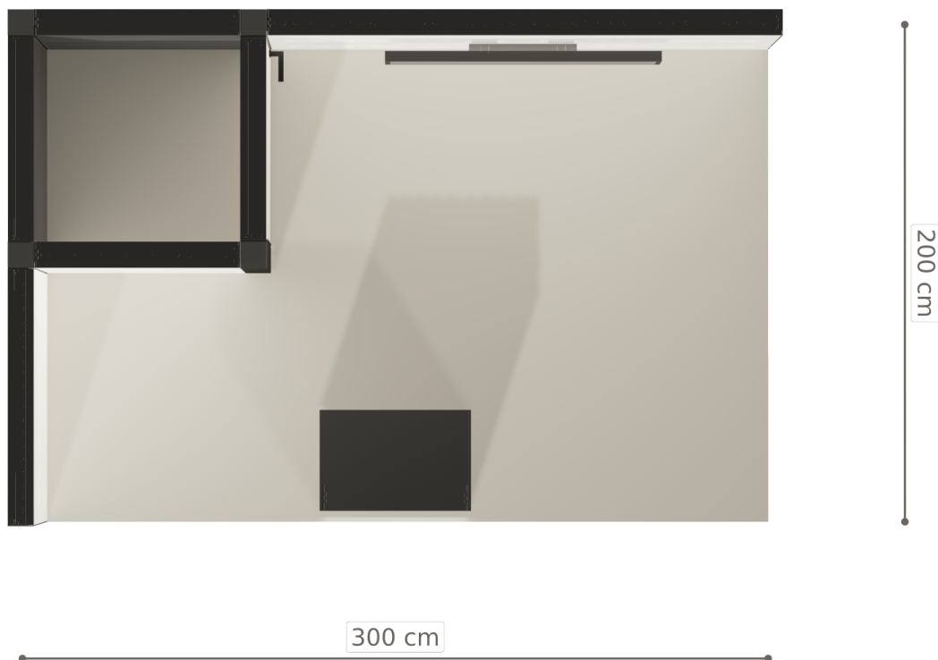
Rzut — szerokości modułów i mebli
