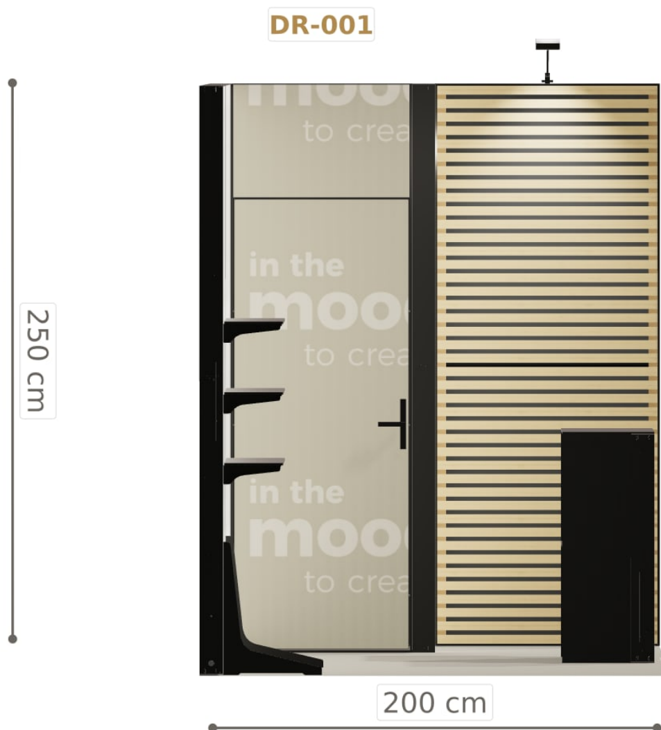
Elewacja z lewej
