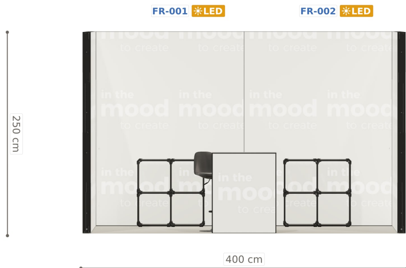
Elewacja ściany tylnej
