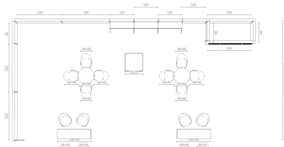
Rzut — szerokości modułów i mebli
