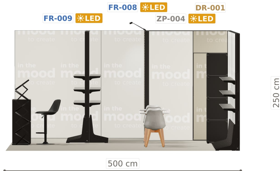
Elewacja ściany lewej
