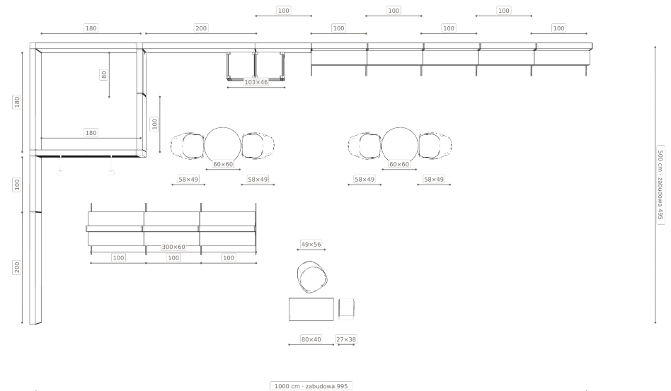
Rzut — szerokości modułów i mebli
