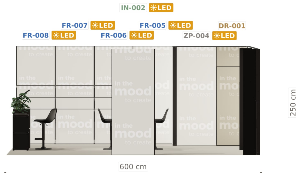
Elewacja ściany lewej
