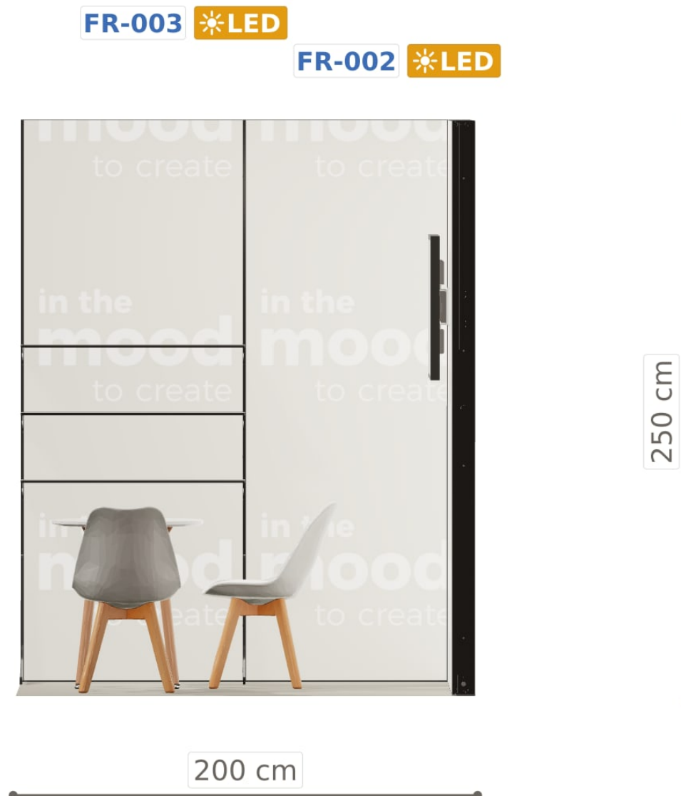
Elewacja ściany lewej
