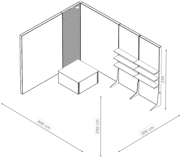
Izometria — wysokości elementów
