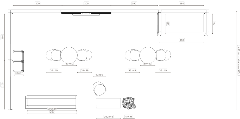
Rzut — szerokości modułów i mebli
