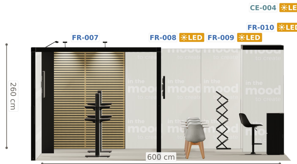
Elewacja ściany prawej
