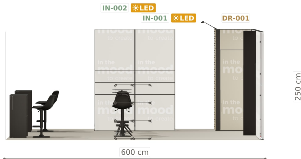
Elewacja z prawej
