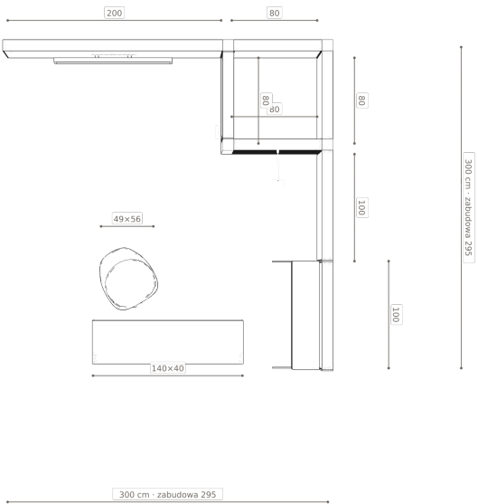
Rzut — szerokości modułów i mebli
