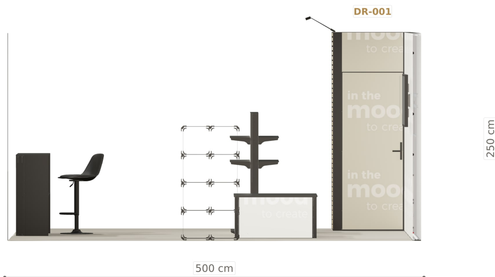
Elewacja z prawej
