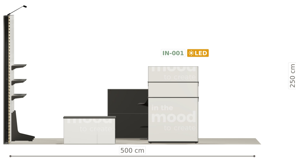
Elewacja od tyłu
