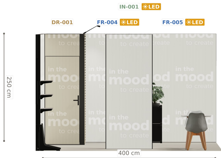
Elewacja ściany prawej
