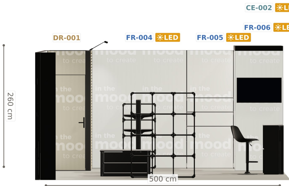
Elewacja ściany prawej
