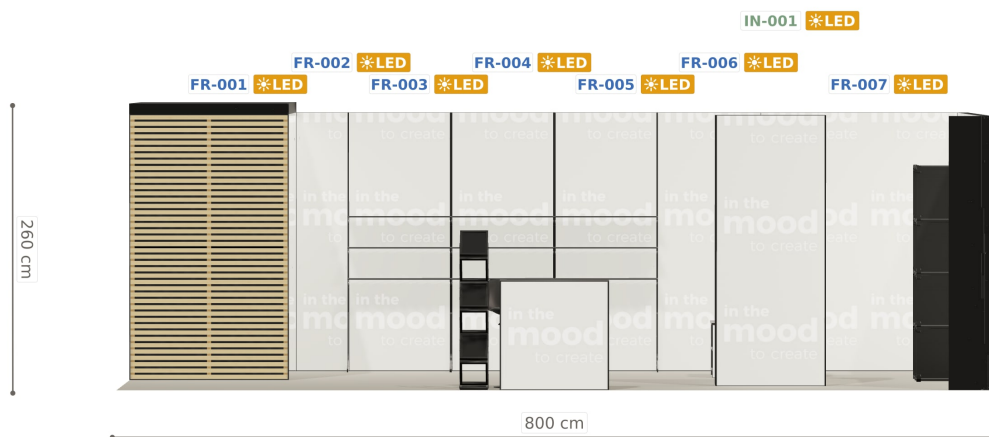
Elewacja ściany tylnej
