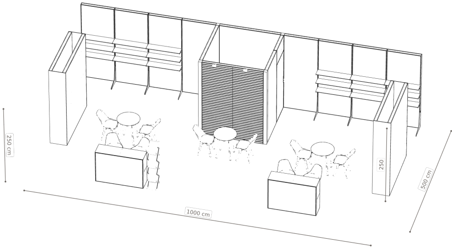
Izometria — wysokości elementów
