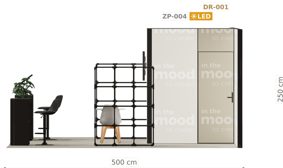
Elewacja z prawej
