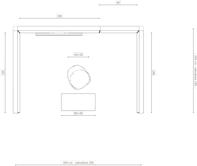
Rzut — szerokości modułów i mebli
